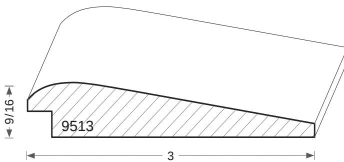
RABBET 1/4 X 1/4
