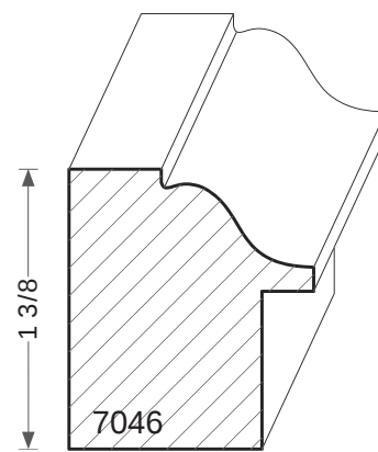
7046 RABBET 1/4 X 3/4
