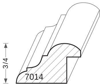
RABBET 1/4 X 1/2
