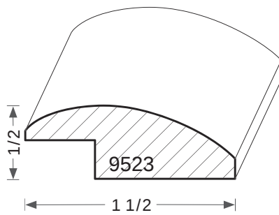
RABBET 1/4 X 1/2
